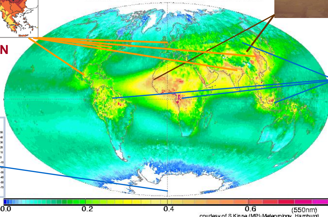
Global Aerosol Optical Depth S. Kinne
